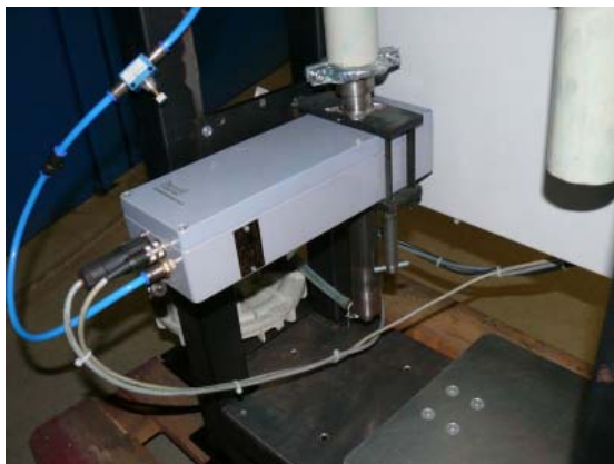
Abb. 4: Der mit Staub beladene Luftstrom wird durch ein Photometer geleitet.
